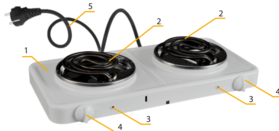
Рис 1. Устройство электроплитки
