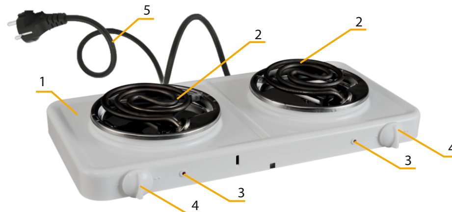
Рис 1. Устройство электроплитки
